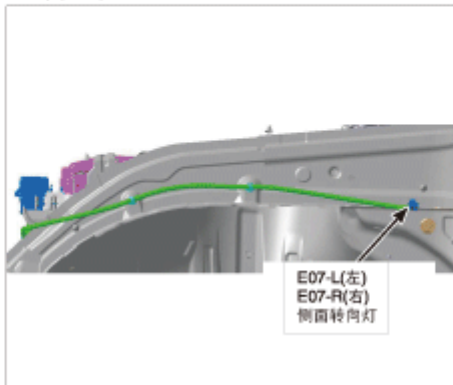
20. 车辆左侧
