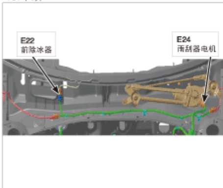
19. 车头
