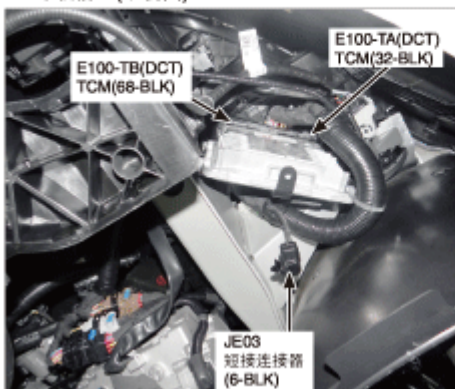
22. 车辆前左(下视图)
