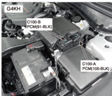
23. 发动机室左侧
